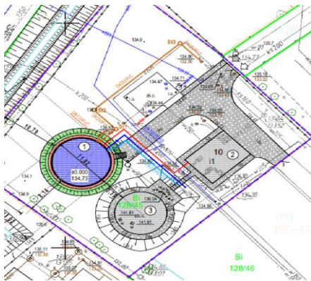
Rys. Projekt zagospodarowania terenu dla budowy zbiornika wody czystej w miejscowości Pietrzykowie.
