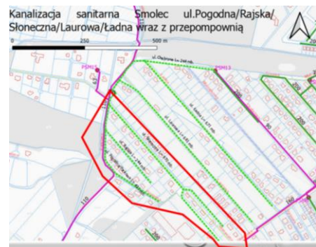
Fot. Kanalizacja sanitarna w miejscowości Smolec w ul. Pogodnej, Parkowej, Rajskiej, Słonecznej, Laurowej i Ładnej.
